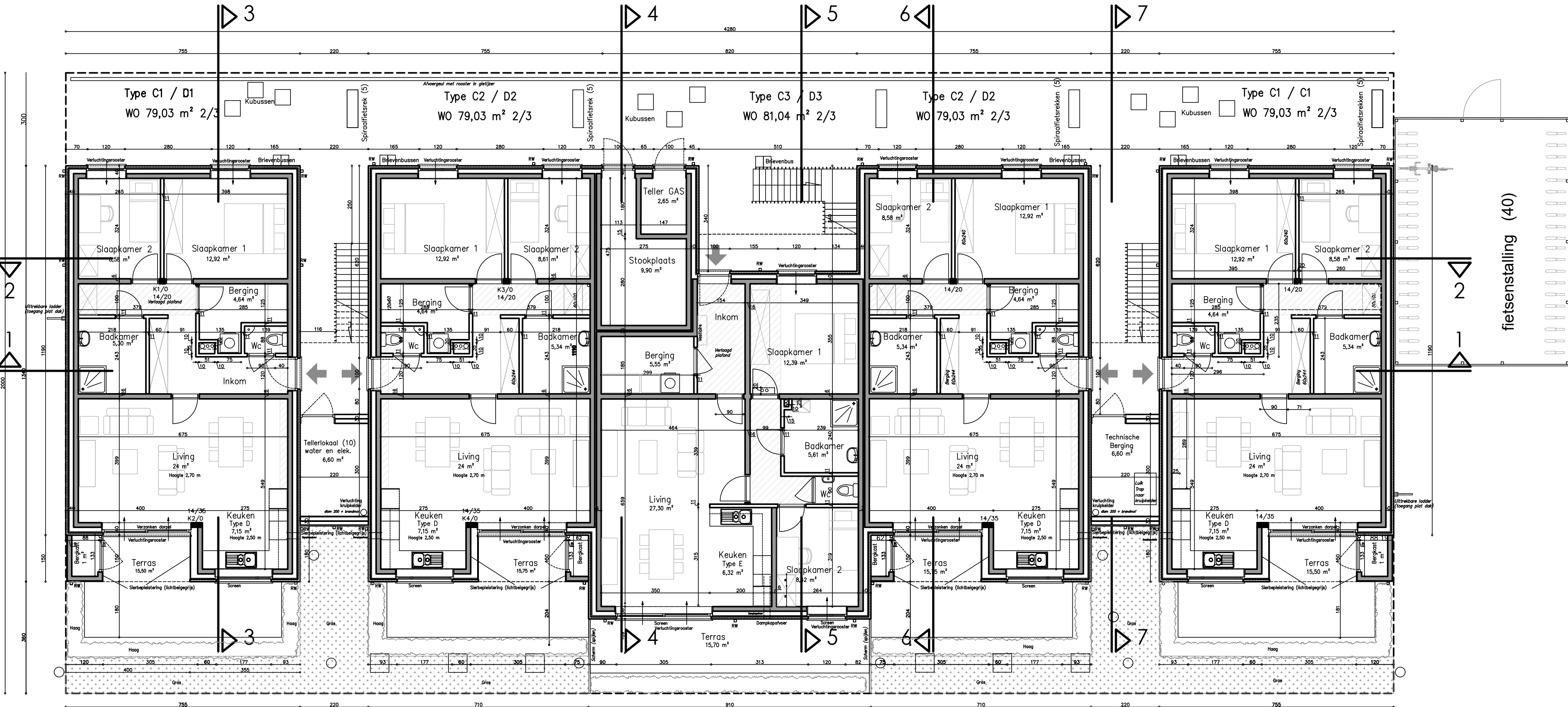
Vloerpeil 0,00 blok C (18.85m)
